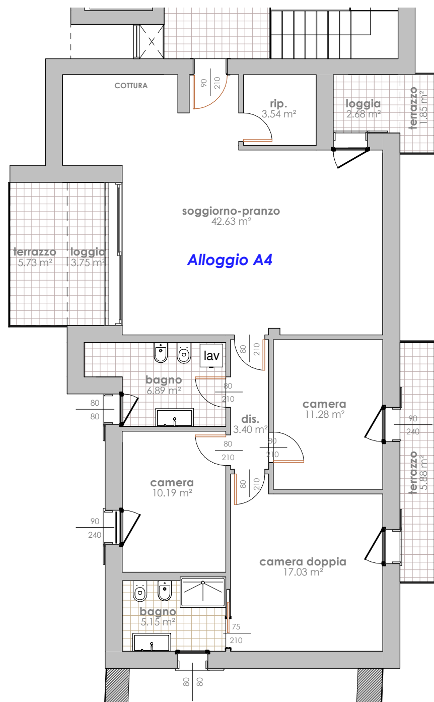
PIANTA PIANO SECONDO sc 1:100
