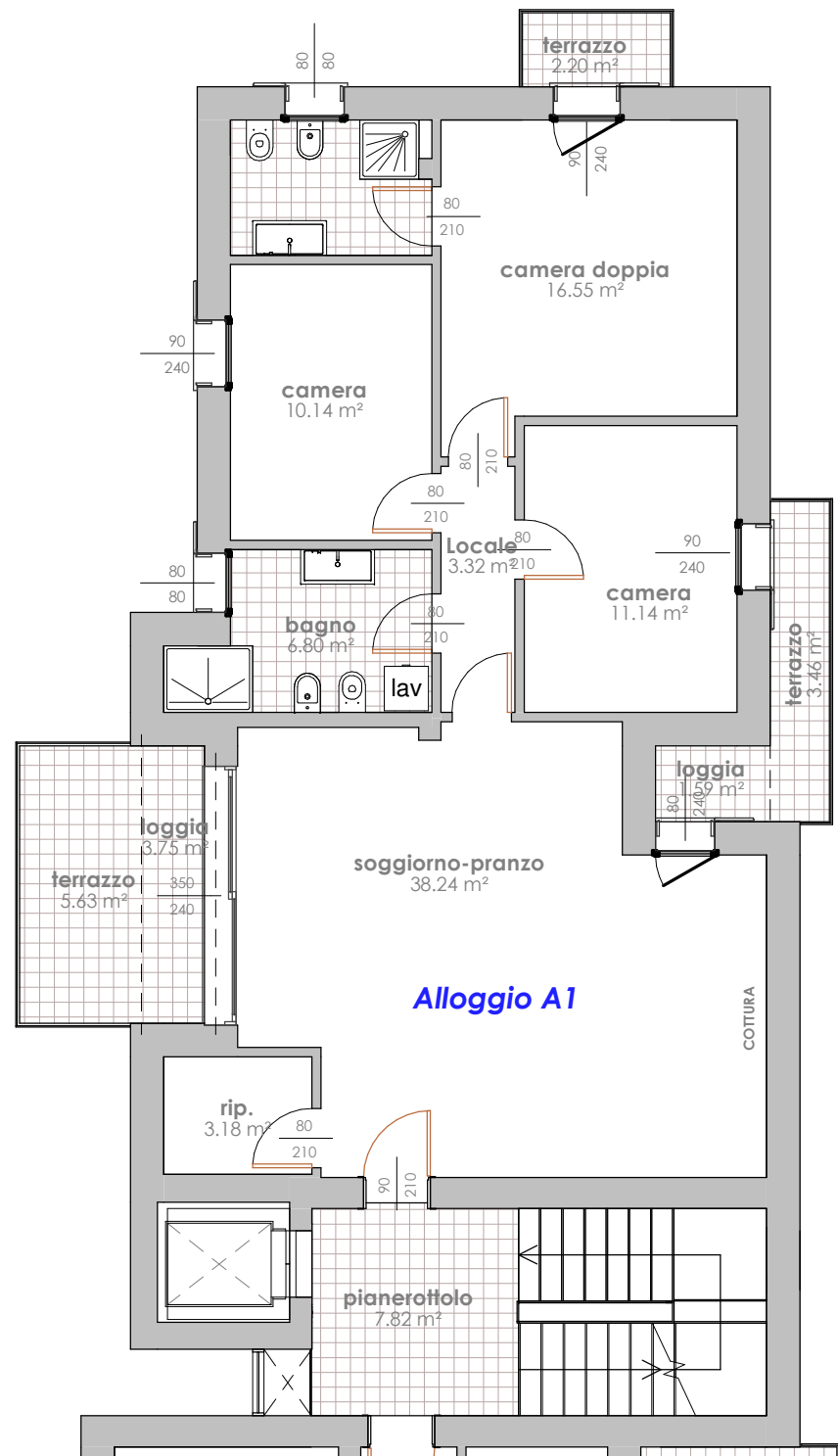
PIANTA PIANO PRIMO sc 1:100
